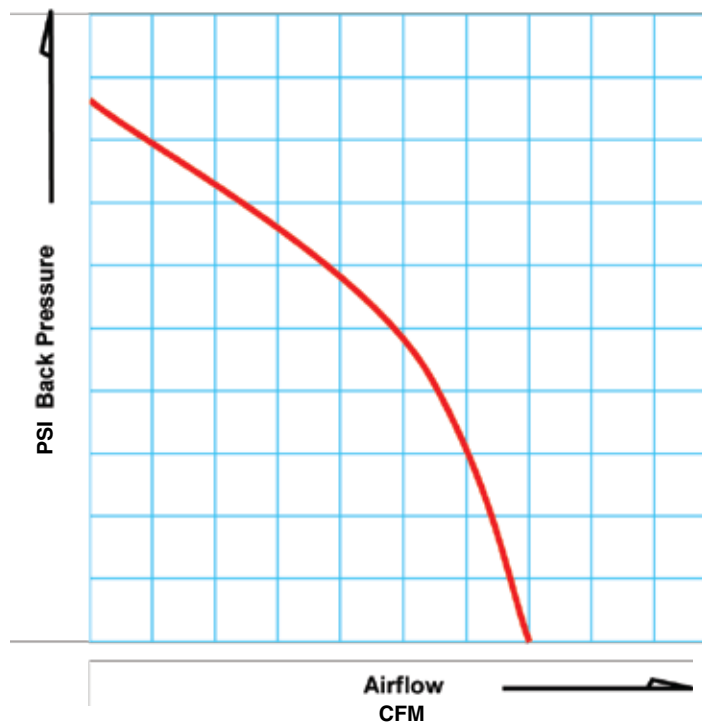
Fan curve.
